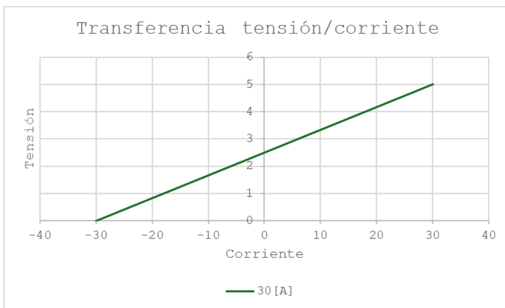
Figura 6 Transferencia corriente/tensión de los sensores (Elaboración Propia)
