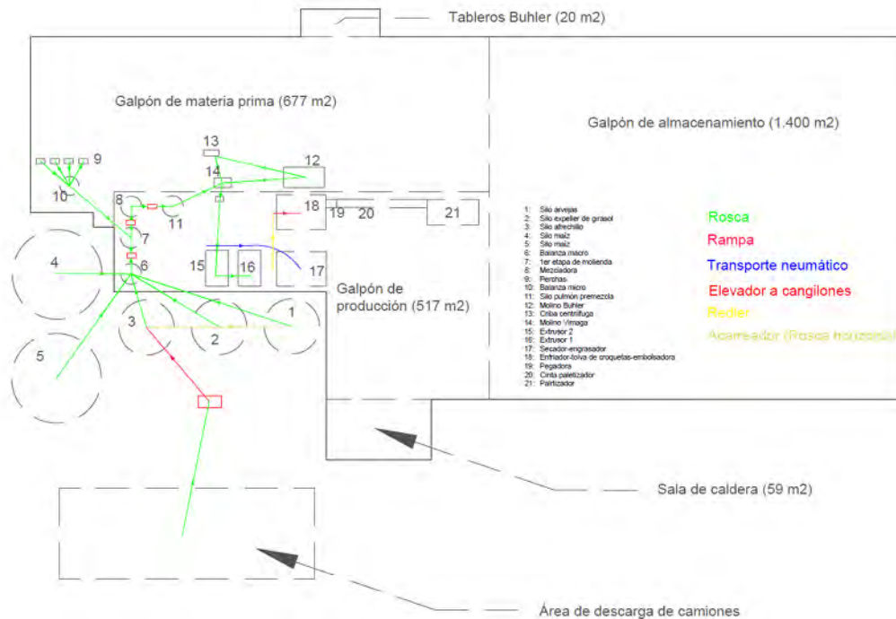
Figura 2 Layout de la planta.
