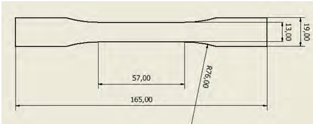
Figura 3 - Cotas utilizadas en mm, según la norma ASTM
