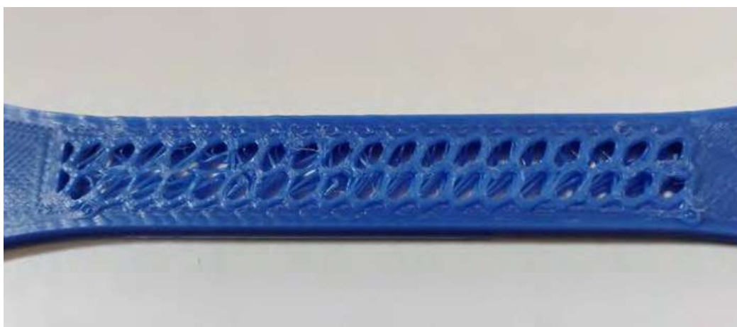
Figura 9 - Primer plano de la zona optimizada de la pieza IV
