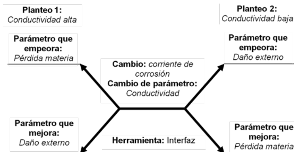
Figura 8. Diagrama de Contradicciones Técnicas sobre el caso del electrodo de puesta a Tierra.
