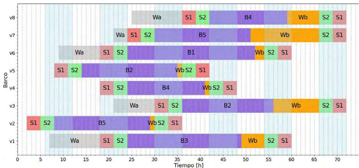
Figura 3 Movimiento de los barcos a lo largo del horizonte de planificación al reducir emisiones.
