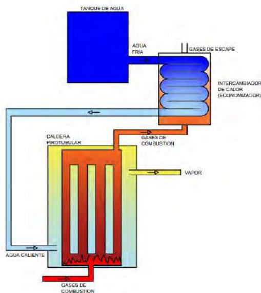
Figura 2 Diagrama esquemático del funcionamiento de una caldera pirotubular equipada con un economizador para la recuperación de calor residual. Referencia: (Elaboración propia)
