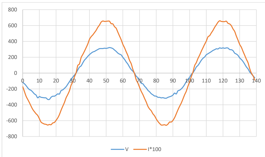
Figura 10 Señales de tensión y corriente con ajuste de fase.
