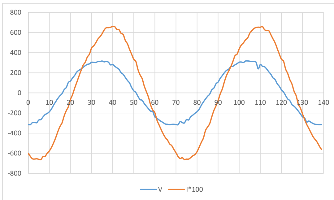
Figura 9 Señales de tensión y corriente sin ajuste de fase.
