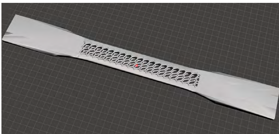
Figura 7 - Modelo en 3D del optimización por Meshmixer
