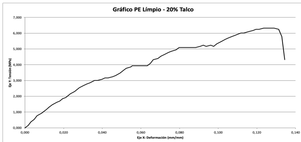
Ensayo tracción caso 2: Probeta PE Limpio - 20% Talco Tensión Máxima (MPa) = 6,323
