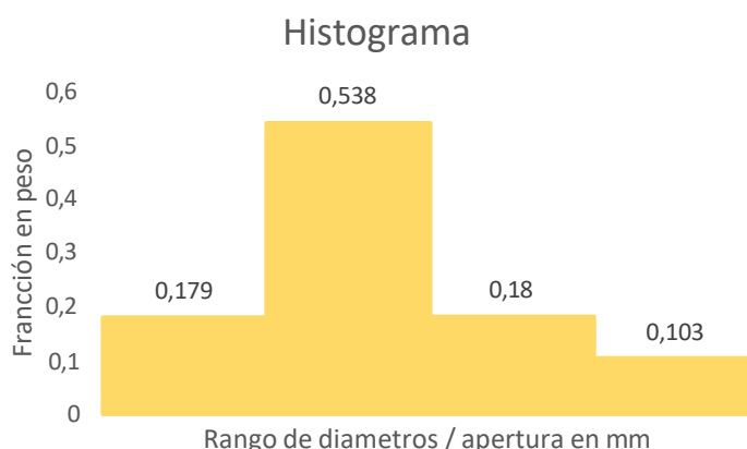
Figura 11: Histograma de distribución granulométrica de la segunda clasificación
