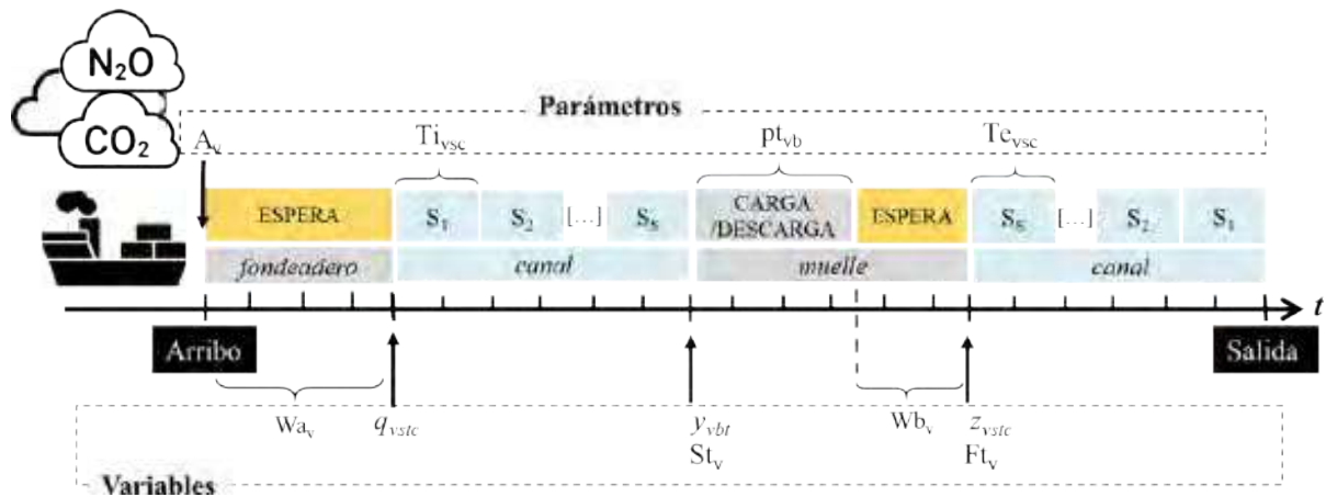
Figura 1 Esquema de las operaciones de los buques en el puerto.
