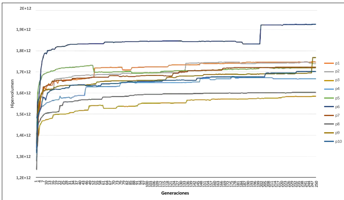
Figura 3 Desempeño de la métrica de hipervolumen para 10 pruebas.
