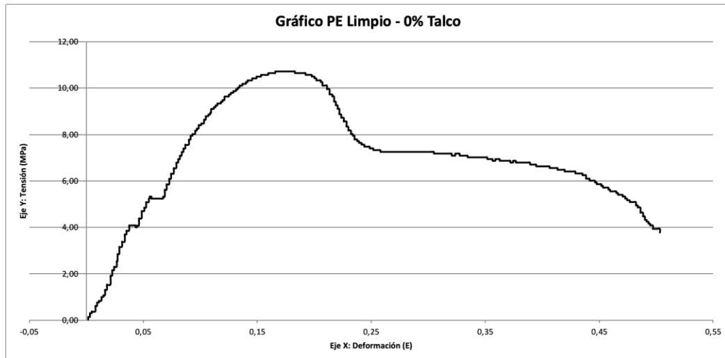
Ensayo tracción caso 1: Probeta PE Limpio - 0% Talco Tensión Máxima (MPa) = 10,725
