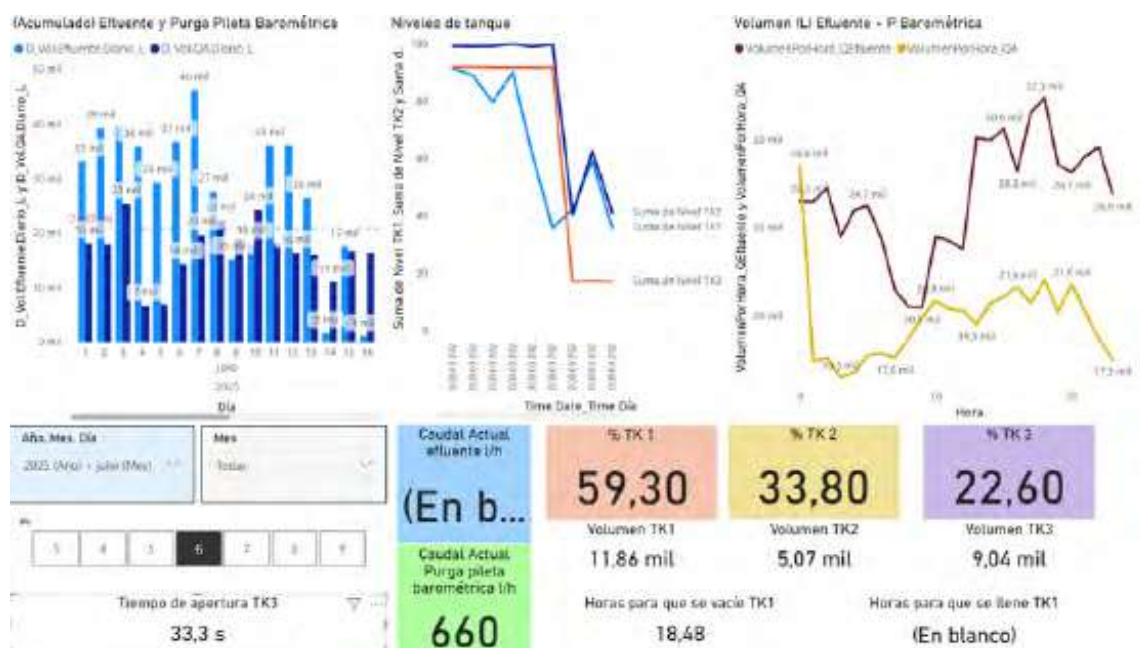
Figura 7. Dinámica operativa de los tanques del sistema de efluentes.
