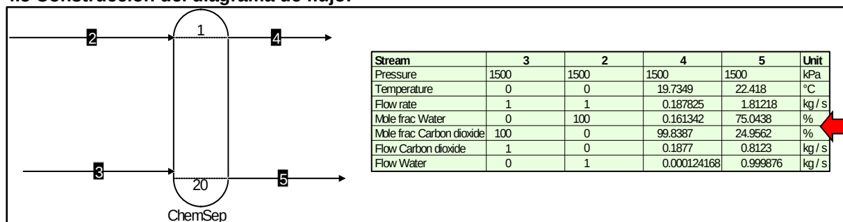
Figura 2. Copia del diagrama de flujo de la columna de absorción con tabla de propiedades COCO
