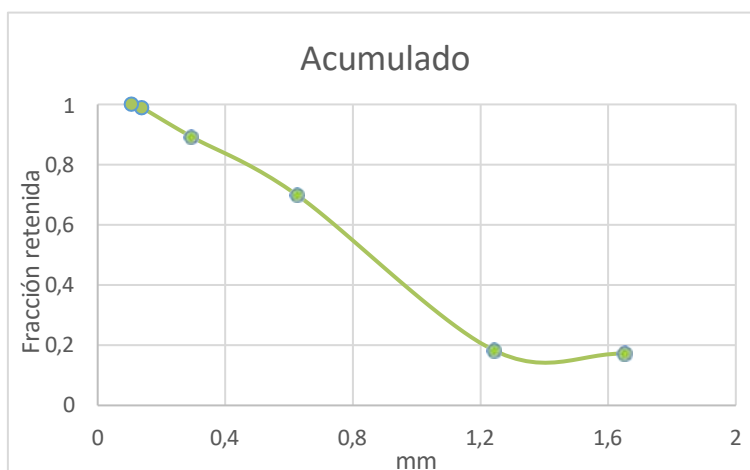
Figura 10: Curva granulométrica de retenido porcentual acumulado
