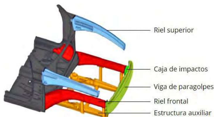
Figura 1 Componentes de la zona delantera del vehículo (Du et al., 2023).
