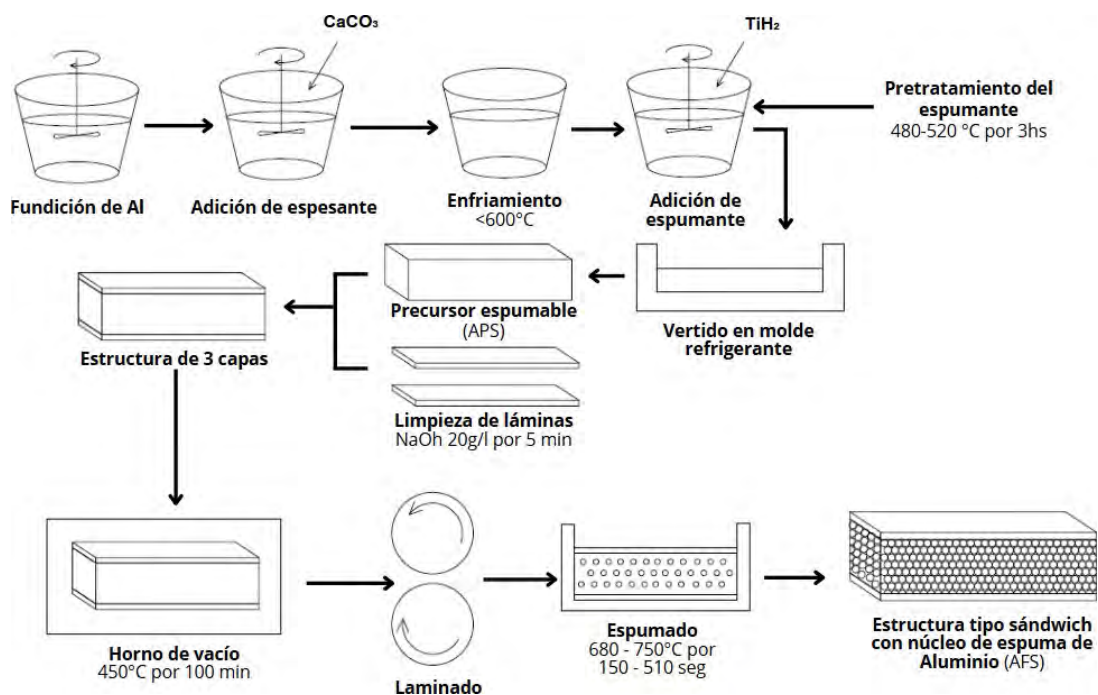
Figura 7 Esquema del proceso de fabricación.
