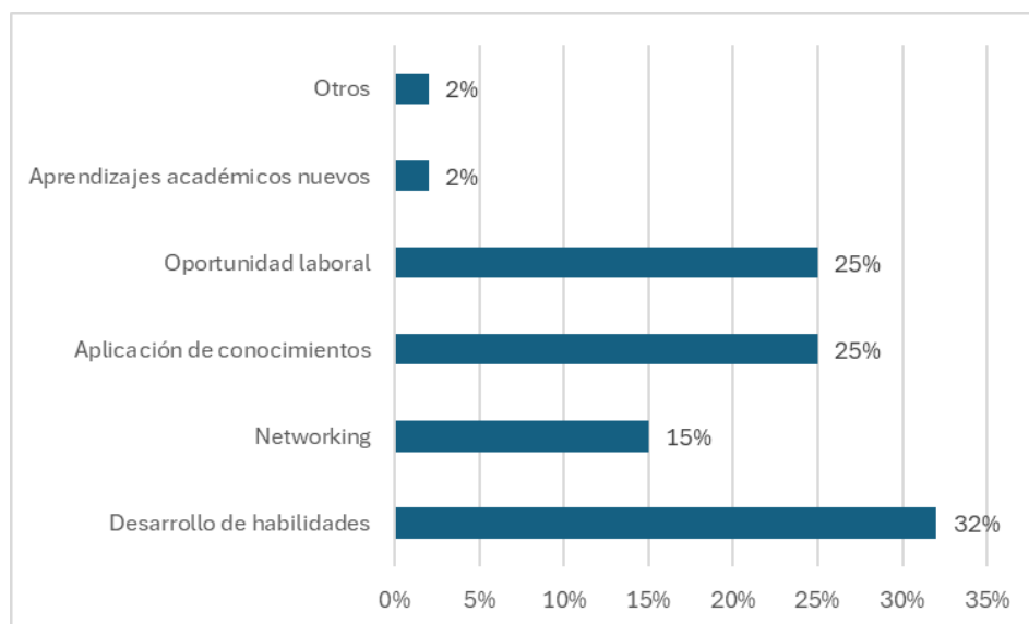
Figura 4 Beneficios percibidos
