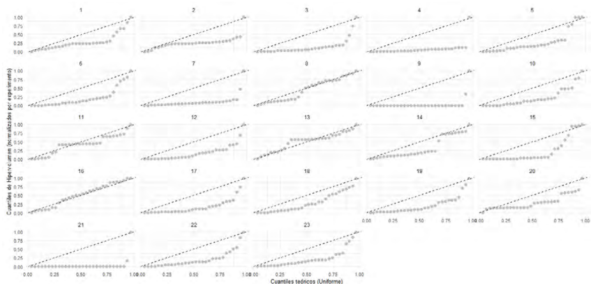
Figura 4 Gráfico Q-Q plot con cuantiles uniformes del hipervolumen para los 23 experimentos del conjunto Nissan.
