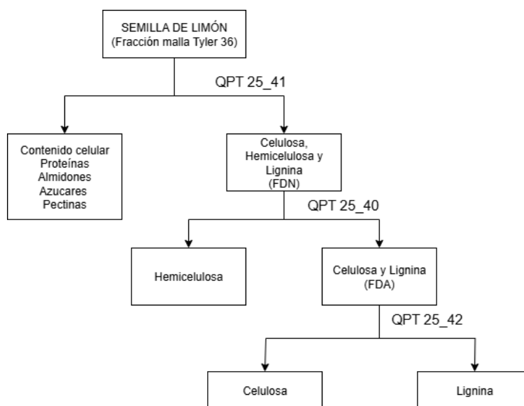
Figura 5: Metodología seguida para la obtención del perfil lignocelulósico.
