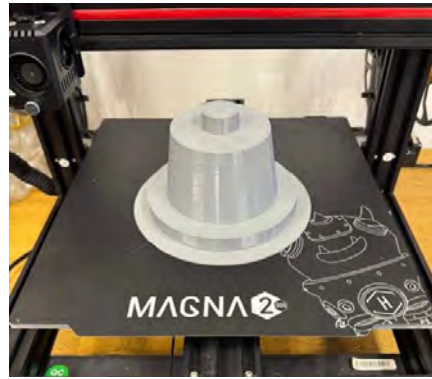
Imagen 1 – Modelo de la pieza A del molde de macetas obtenida mediante impresión 3D
