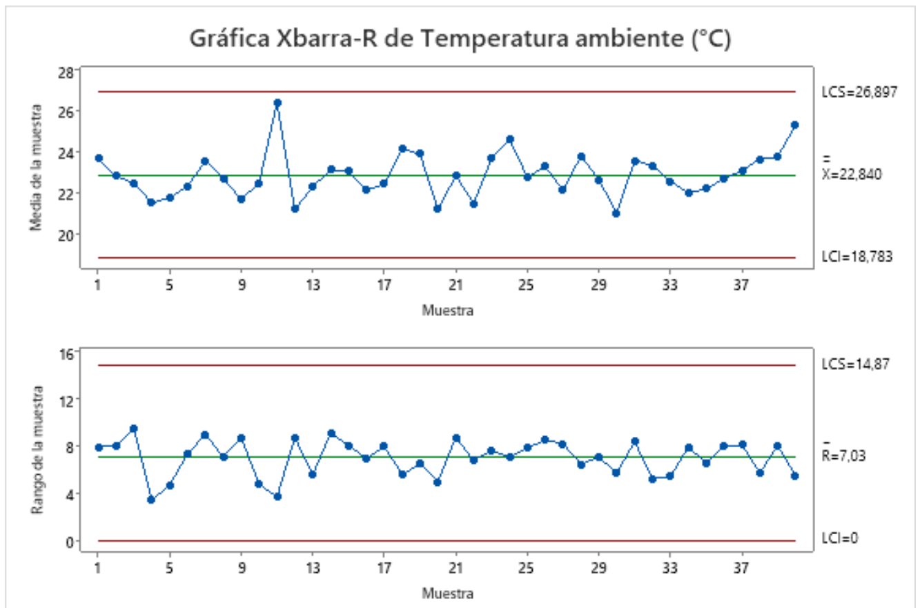
Figura 5: Gráfica de medias y Gráfica de rangos
