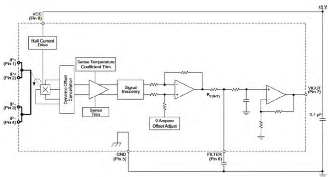
Figura 7 Diagrama del sensor de Corriente (Allegro Microsystems, 2024)
