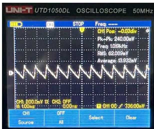
Figura 2 Señal de alimentación usando fuente conmutada de 220 VAC a 5 VDC.
