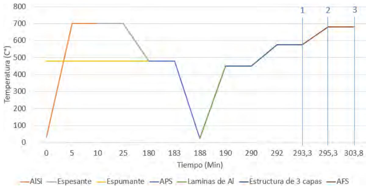
Figura 8 Esquema de temperatura y tiempos del proceso.
