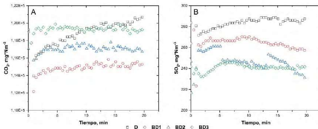
Figura 4 Diagrama de gases: A) emisiones gaseosas de CO 2 y B) emisiones gaseosas de SO 2
