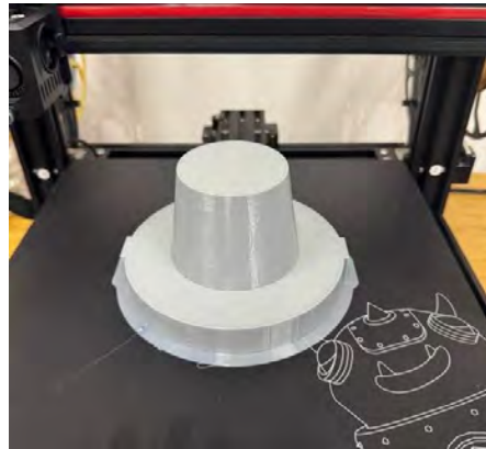
Imagen 2 – Modelo de la pieza B del molde de macetas obtenida mediante impresión 3D
