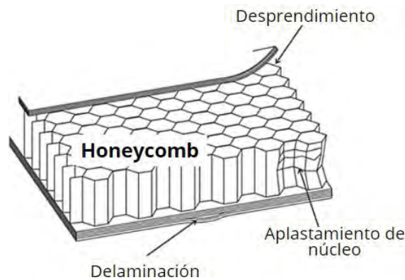
Figura 4 Modos de falla de una estructura con núcleo Honeycomb (Girolamo et al., 2018).
