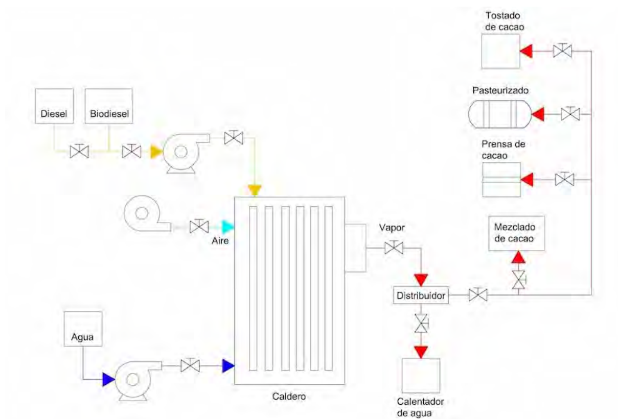
Figura 1 Diagrama esquemático del sistema de generación de vapor, y la operación con la mezcla de biodiesel – diésel.
