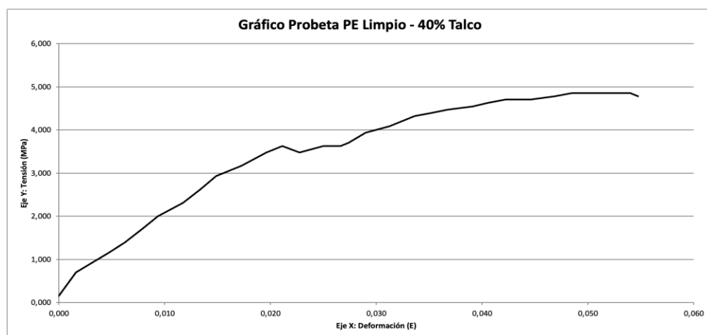
Ensayo tracción caso 3: Probeta PE Limpio - 40% Talco Tensión Máxima (MPa) = 4,857
