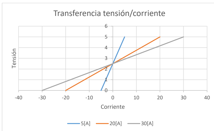
Figura 1 Transferencia corriente/tensión de los sensores ACS712.
