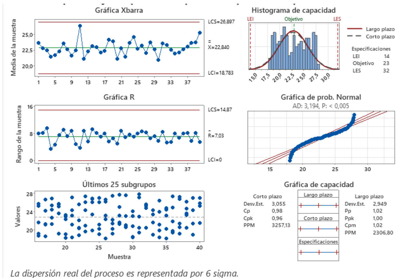
Figura 6 : Informe del Capability Sixpack del proceso para Temperatura ambiente (°C)
