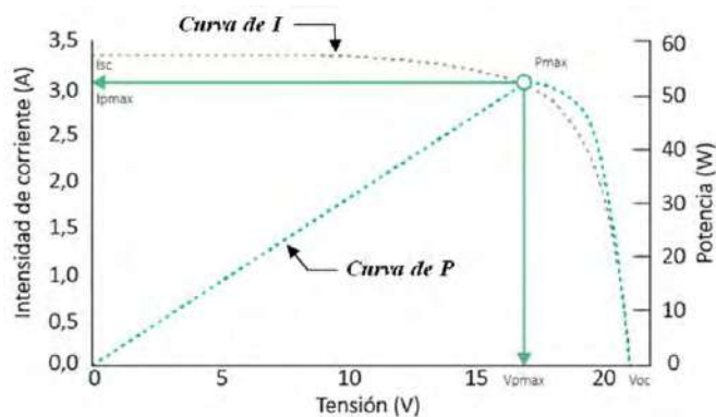
Figura 6: Gráfico de Intensidad en fusión de la Tensión y Potencia
