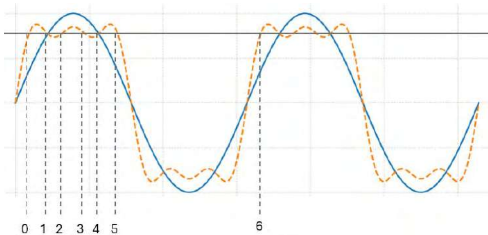
Figura 6 Cruces de señal por valor fijo de tensión en senoidal con distorsión armónica.
