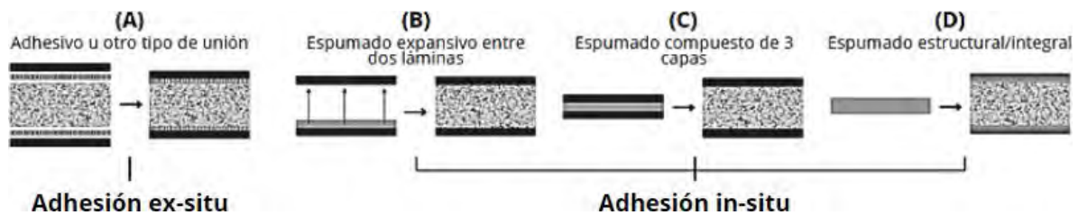
Figura 6 Tipos de adhesión (Banhart & Seeliger, 2008).
