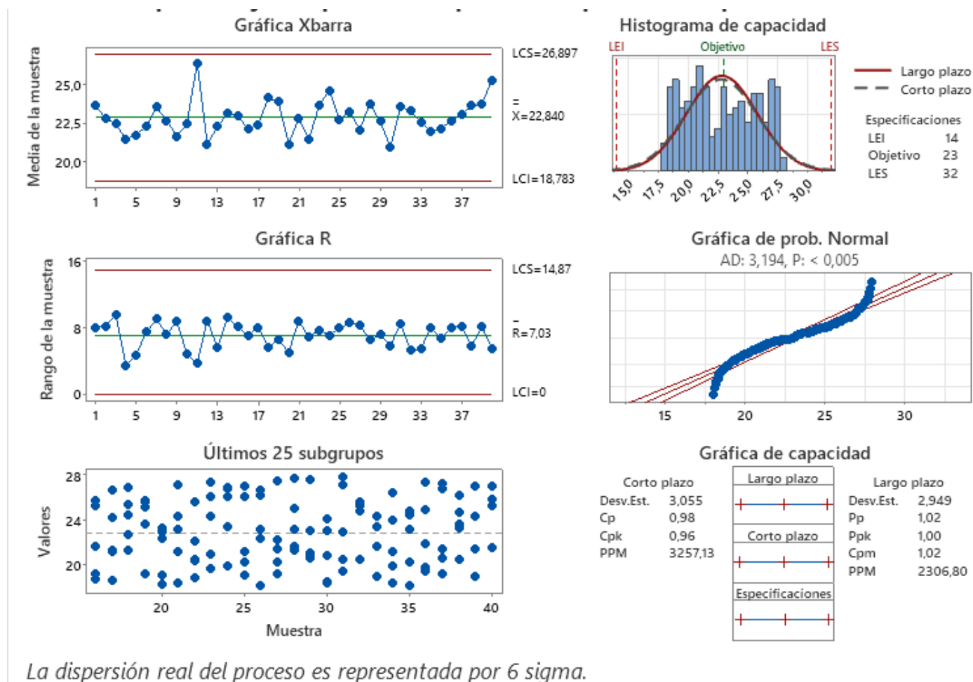
Figura 6 : Informe del Capability Sixpack del proceso para Temperatura ambiente ( ^{\circ}\text{C} )
