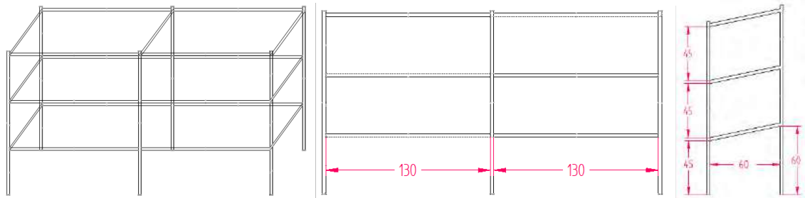
Figura 2. Diseño de la estantería medida en cm (de izquierda a derecha: Estantería, vista frontal, vista lateral)
