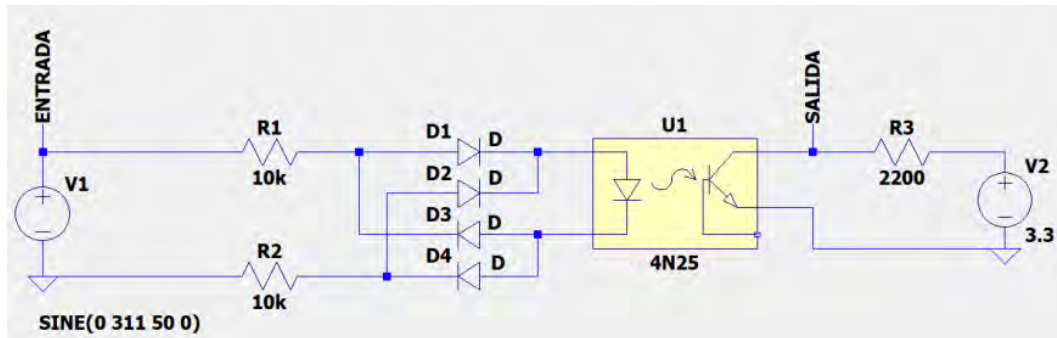
Figura 7 Circuito esquemático de detector de cruce por cero.
