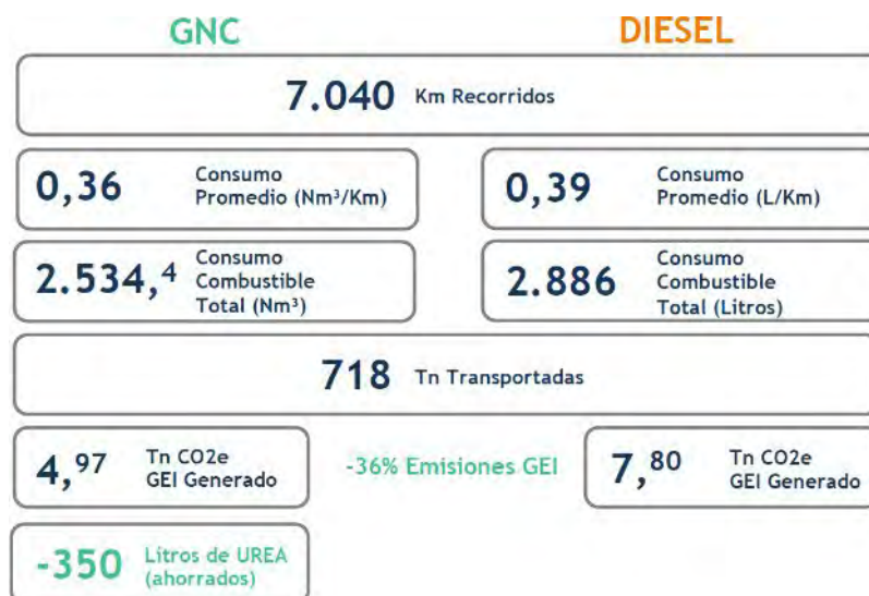
Figura 2 Resultados tras 60 días de utilización de unidad impulsada a GNC vs unidad promedio Diesel. Fuente: Ilustración propia
