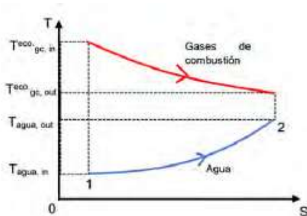
Figura 1 Curva típica de los gases de combustión y del agua de alimentación, posterior a la instalación de un economizador en el sistema de caldera. Referencia (Elaboración propia)
