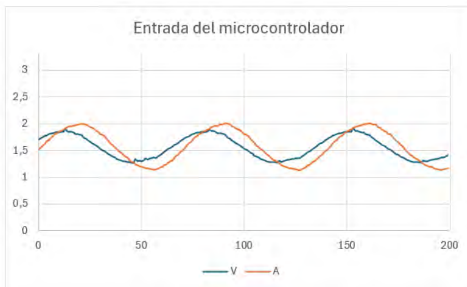
Figura 4 Señales brindadas por los sensores usando regulador lineal 7805.
