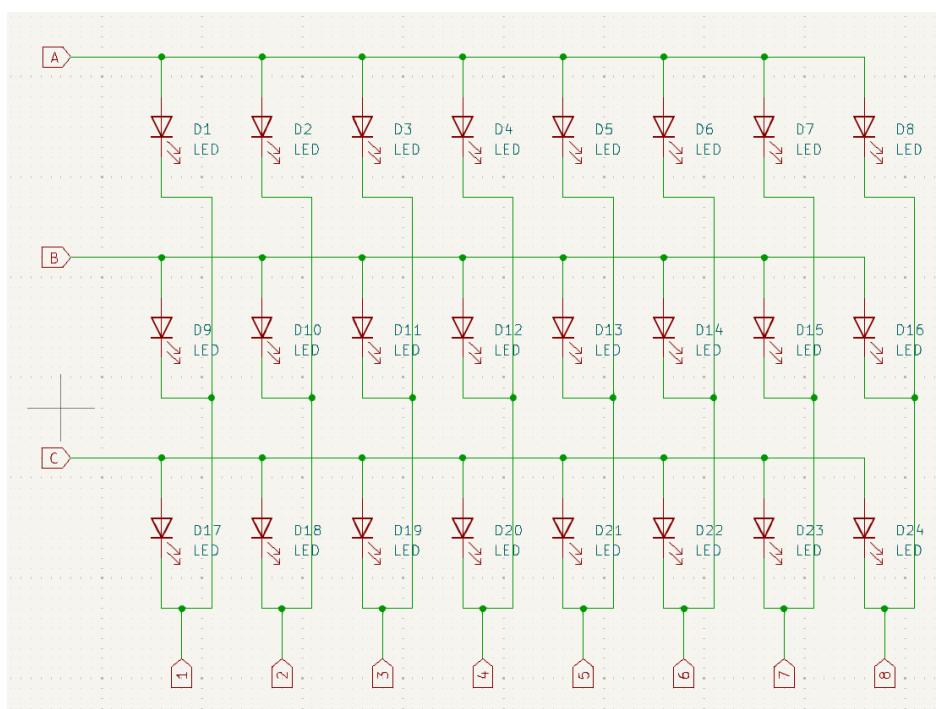
Figura 4. Esquema eléctrico de la matriz.
