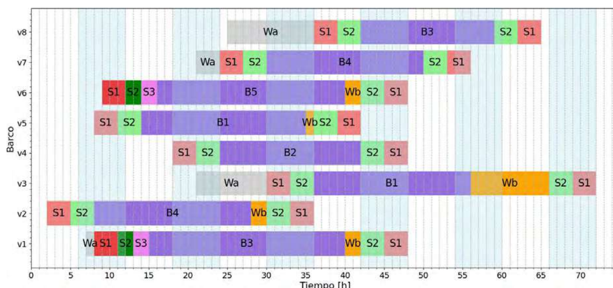
Figura 2 Movimiento de los barcos a lo largo del horizonte de planificación al minimizar costos.
