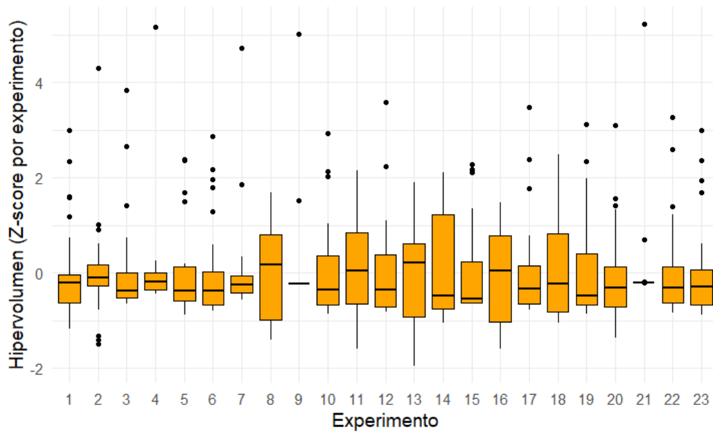
Figura 3 Gráfico boxplot del hipervolumen estandarizado por experimento para los 23 experimentos del conjunto Nissan.
