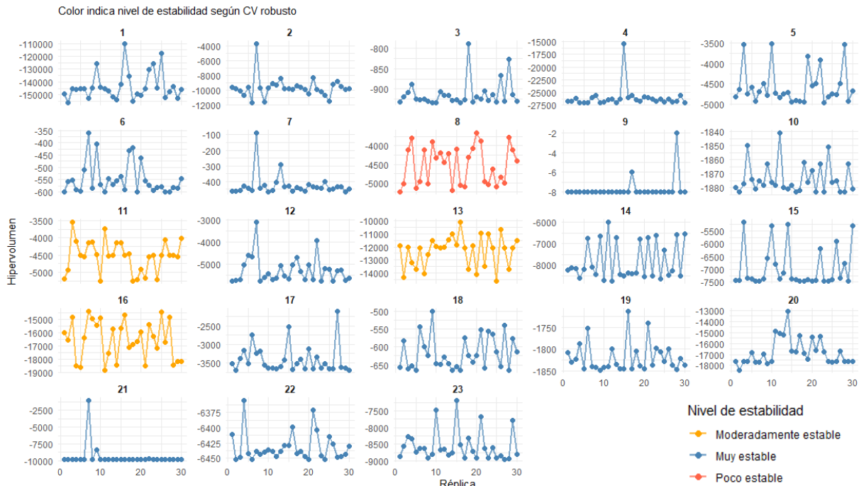
Figura 1 Variación del hipervolumen por réplica para los 23 experimentos del conjunto Nissan.
