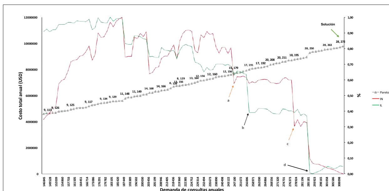
Figura 4 Frente de Pareto demanda-costo e inequidades en cobertura y carga laboral.
