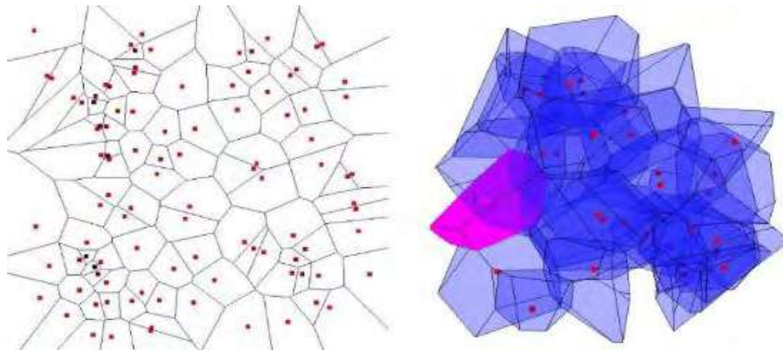
Figura 2 - Diagrama de Voronoi en 2D (izquierda) y 3D (derecha) Fuente: Ying et al., 2015
