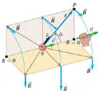
Figura 10: Campo magnético “B” producido por una carga en movimiento.
