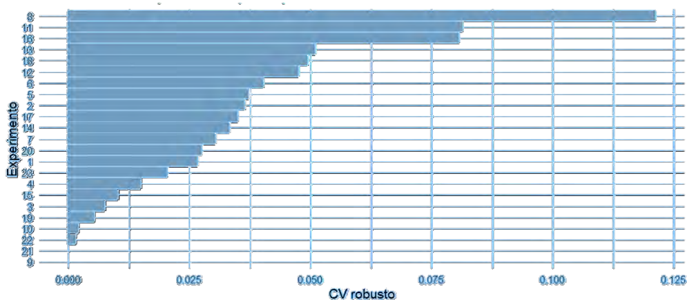
Figura 2 CV_robusto del hipervolumen calculado para los 23 experimentos del conjunto Nissan.
