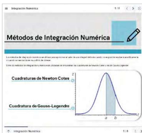
Figura 1. Explicación teórica de los métodos numéricos
