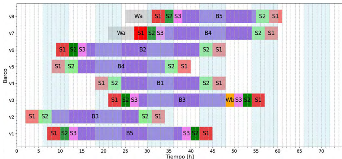
Figura 4 Movimiento de los barcos a lo largo del horizonte de planificación al minimizar tiempo.
