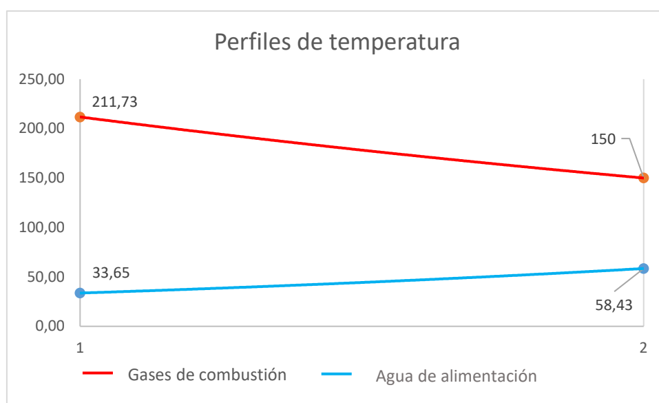
Figura 6 Diagrama de los perfiles de temperatura de los gases de combustión y del agua de alimentación, posterior a la instalación de un economizador en el sistema de caldera. Referencia: (Elaboración propia)
