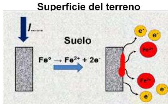
Figura 7. Esquema gráfico del electrodo de puesta a Tierra.
