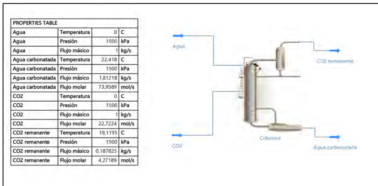
Figura 1. Copia del diagrama de flujo de la columna de absorción con tabla de propiedades DWSIM
