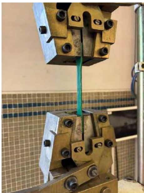
Imagen 24 - Ensayo de tracción
