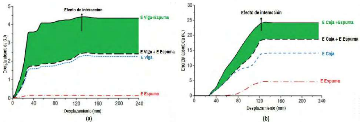
Figura 2 Efecto de interacción en la absorción de energía en estructuras rellenas de espuma: (a) viga de paragolpes relleno de espuma y (b) caja de impacto rellena de espuma (Li et al., 2017).
