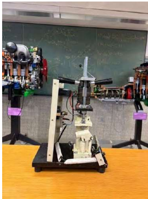
Imagen 23 - Inyectora derivada de inclusora metalográfica, vista lateral
