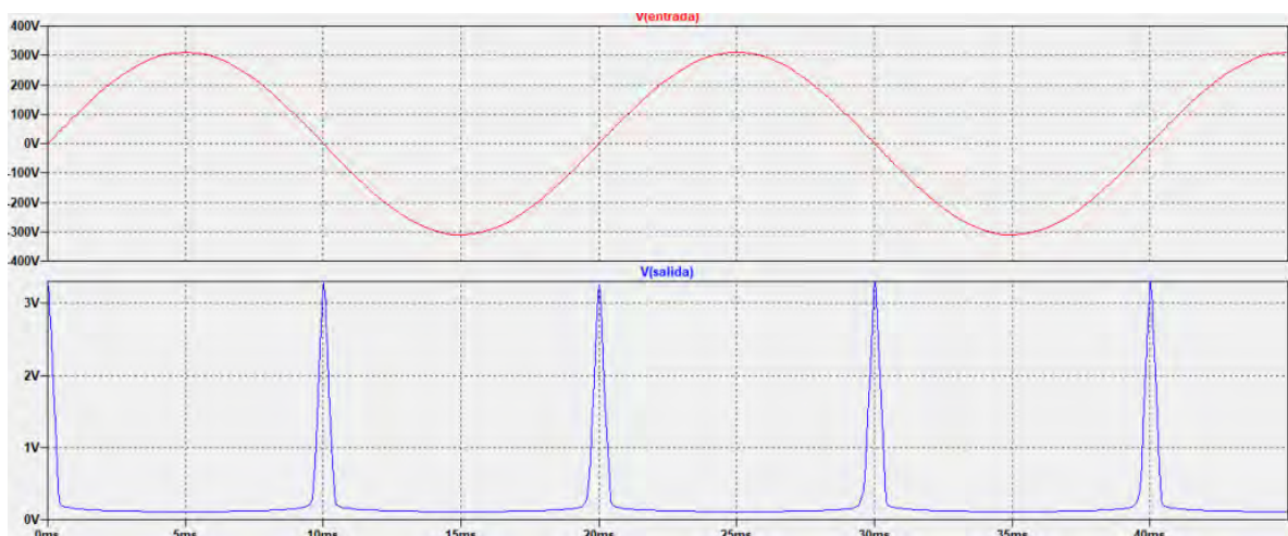
Figura 8 Simulación de señales de detector de cruce por cero.
