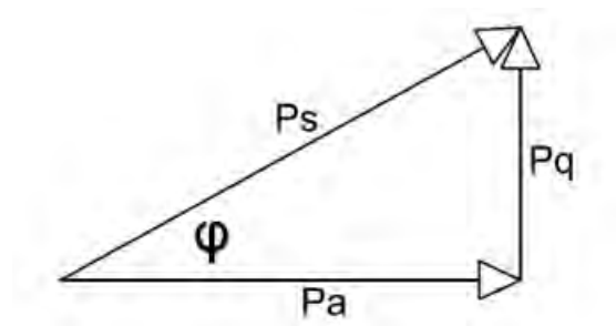
Figura 3 Triángulo de potencias (Elaboración Propia)
