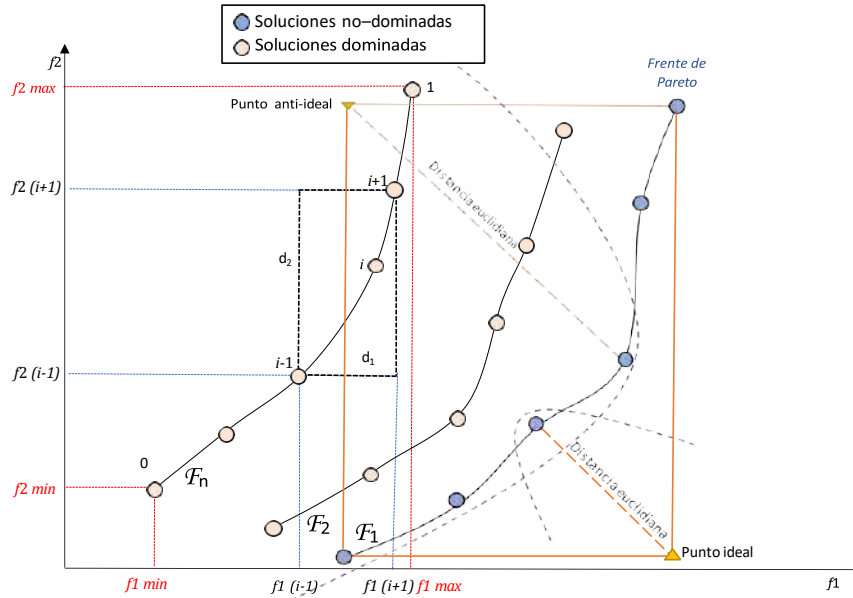
Figura 2 Frente de Pareto del NSGA-II y distancia de apilamiento.
