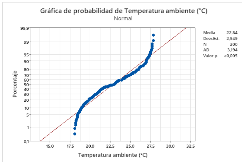
Figura 4: Gráfica de probabilidad de la variable Temperatura ambiente
