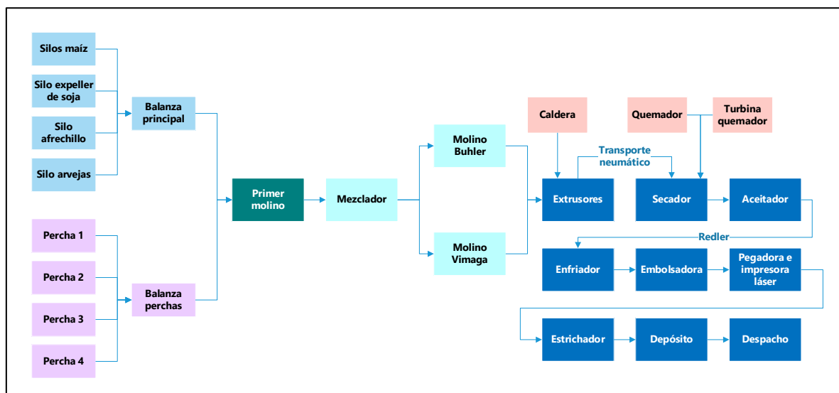
Figura 1 Flujo de procesos de la planta.
