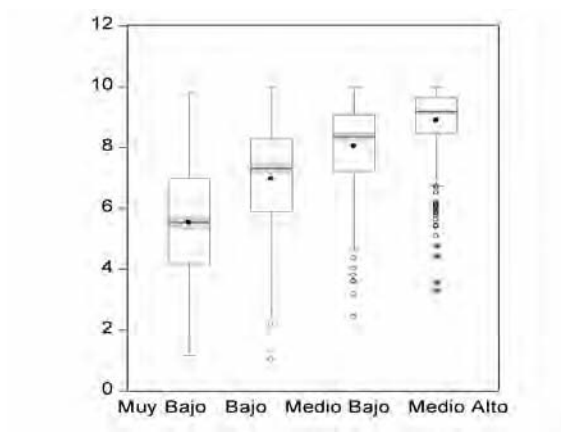
GRÁFICO 18b: Boxplot de las calificaciones del ICV según estrato socioeconómico. 2004
