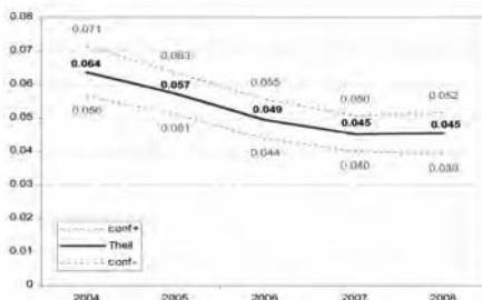
GRÁFICO A.2: Coeficiente de Theil e intervalos de confianza.
